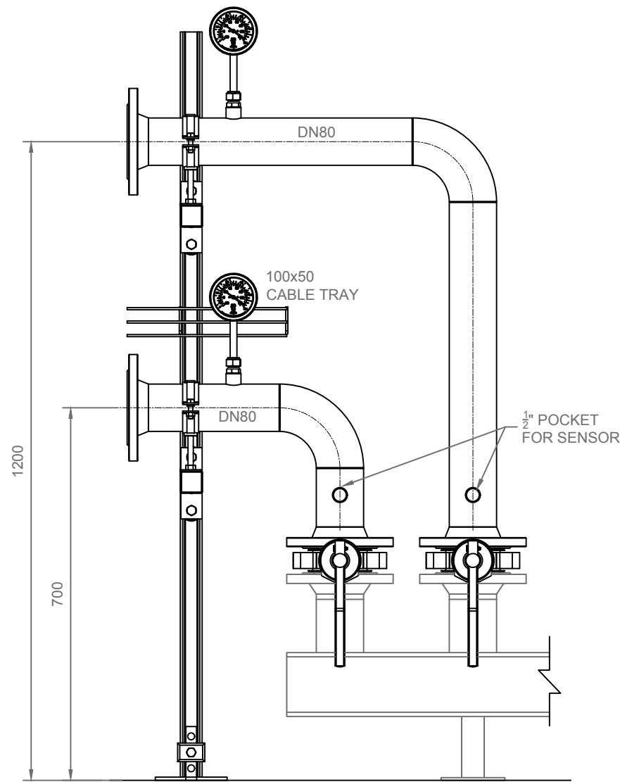
ELEVATION
