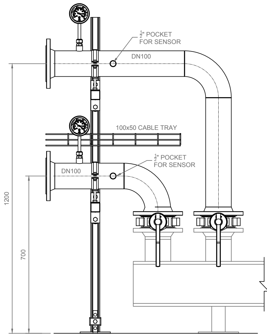
ELEVATION
