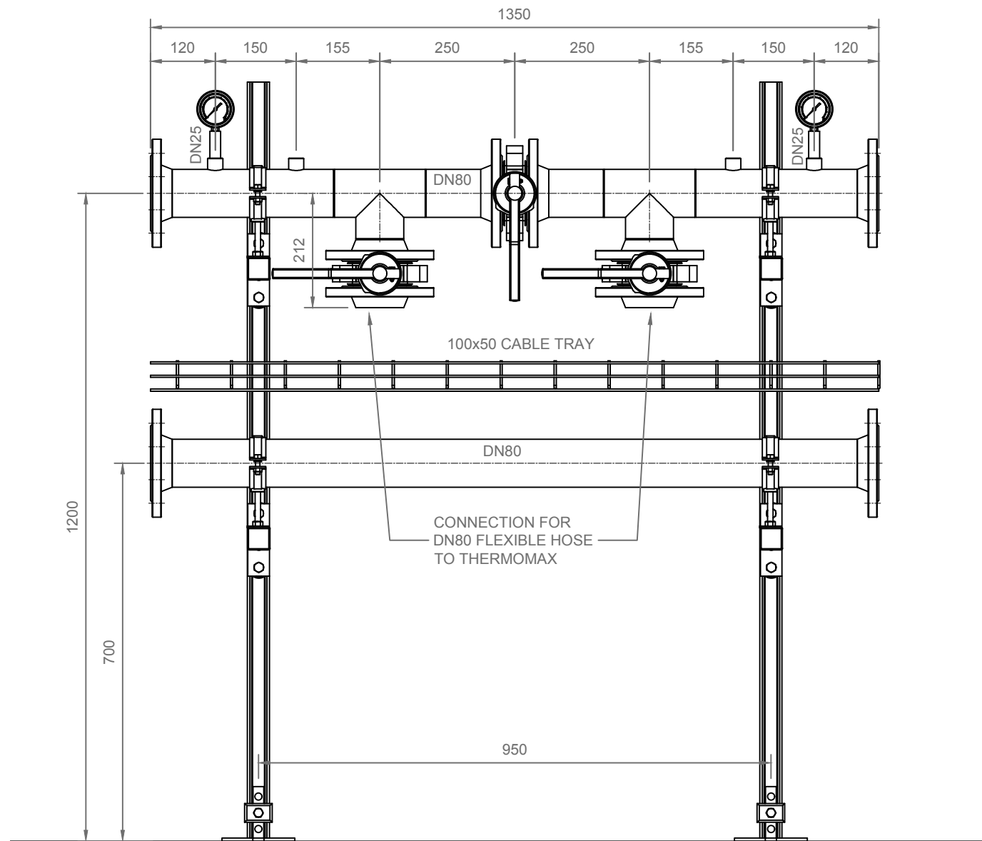
ELEVATION
